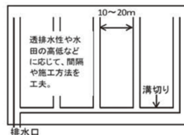
図 3 溝切りの施工方法
