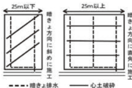
図 2 心土破碎の施工方法
